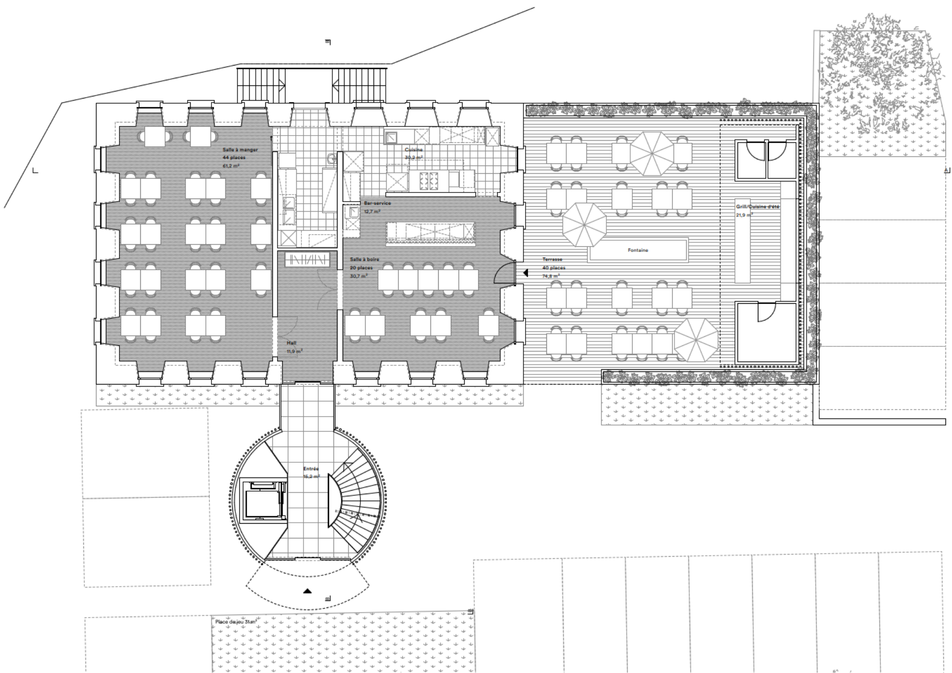
Plan rez-de-chaussée 1:100
